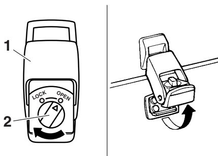
1 Trinco do capot
