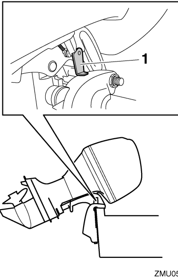
1. Ankipf-Arretierungshebel
