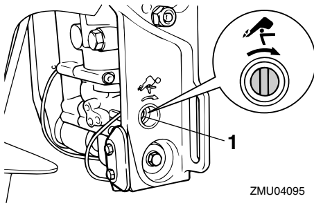
1. Parafuso da válvula manual
