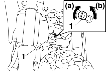
1. Leerlauf­einstellschraube
