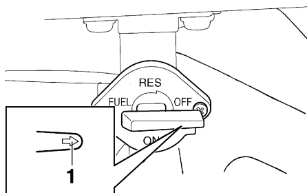
1. Pfeilmarkierung über "OFF" platziert
