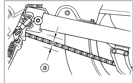
a. Kettendurchhang
