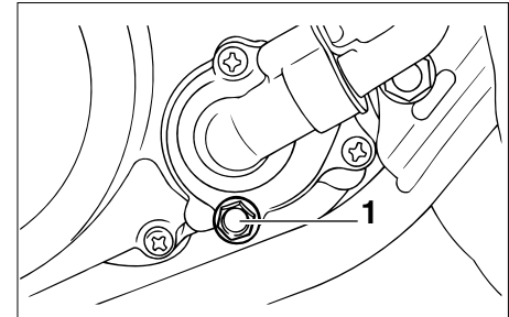
1. Kühlfüssigkeits-Ablafschraube
