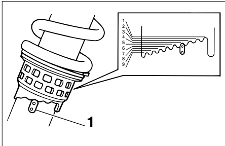
1. Gegenmarkierung
