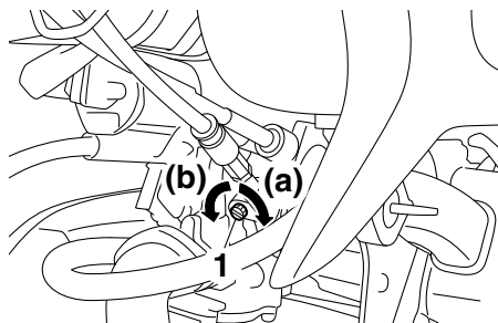
1. LeerlaufEinstellschraube
