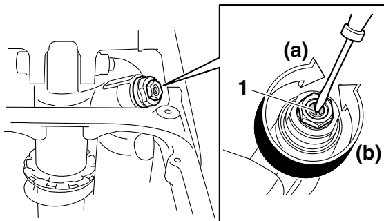
1. Vis de réglage de la force d'amortissement à la compression lente
