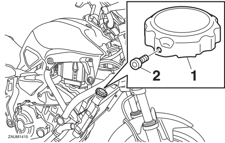
1. Tampa do radiador 2. Parafuso retentor da tampa do radiador
