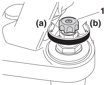
1. Botão ajustador da força amortecedora de recuo
