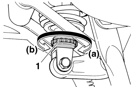
1. Botão ajustador da força amortecedora de recuo
