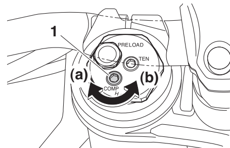
1. Cavilha ajustadora da força amortecedora de compressão
