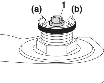
1. Parafuso ajustador da força amortecedora de recuo
