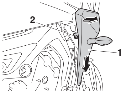
1. Painel A 2. Fixador rápido (tipo parafuso)
