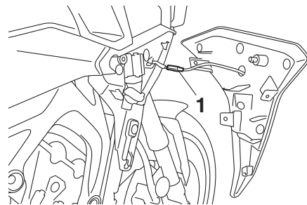
1. Acoplador do fio do sinal de mudança de direção
