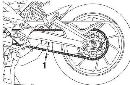
1. Spanning aandrijfketting
