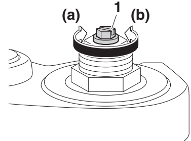
1. Parafuso ajustador da força amortecedora de recuo
