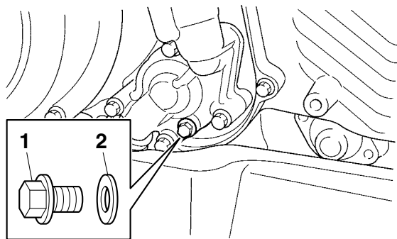
1. Vis de vidange du liquide de refroidissement 2. Joint
