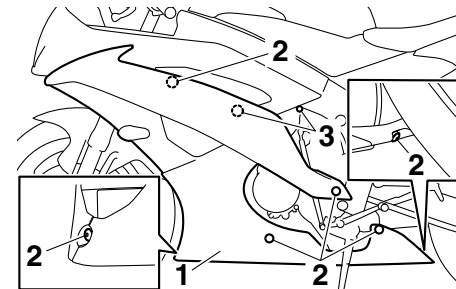
1. Carenagem A 2. Cavilha 3. Fixador rápido
