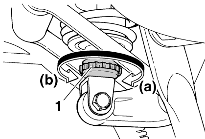
1. Botão ajustador da força amortecedora de recuo
