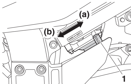
1. Alavanca ajustadora de pré-carga da mola
