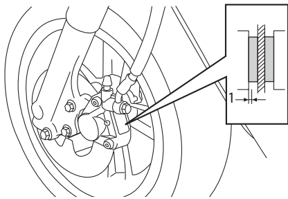
1. Pinça do travão dianteiro
