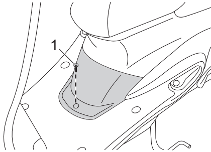
1. Parafuso de fixação do painel
